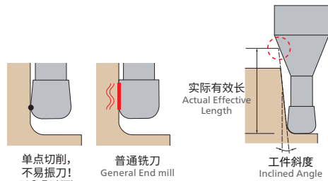
单点切削, 不易振刀! (φ2.5以下) Suppress chattering by point milling (Dia.~2.5)
